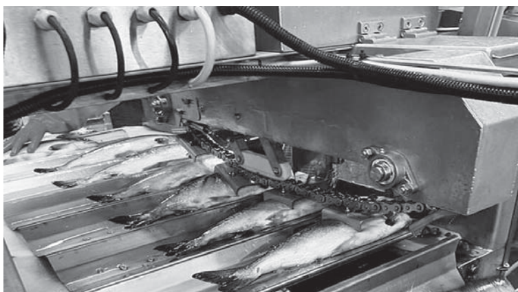
Линия по переработке лосося производства ДРТЦ
