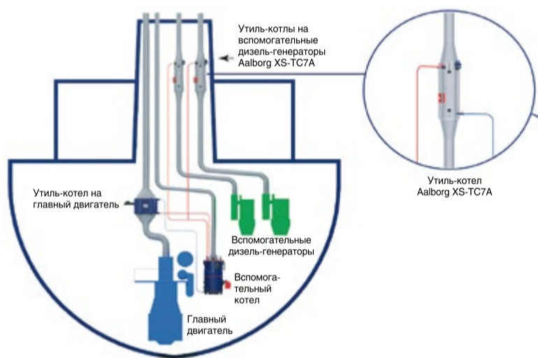
Схема размещения утиль-котлов на судне
